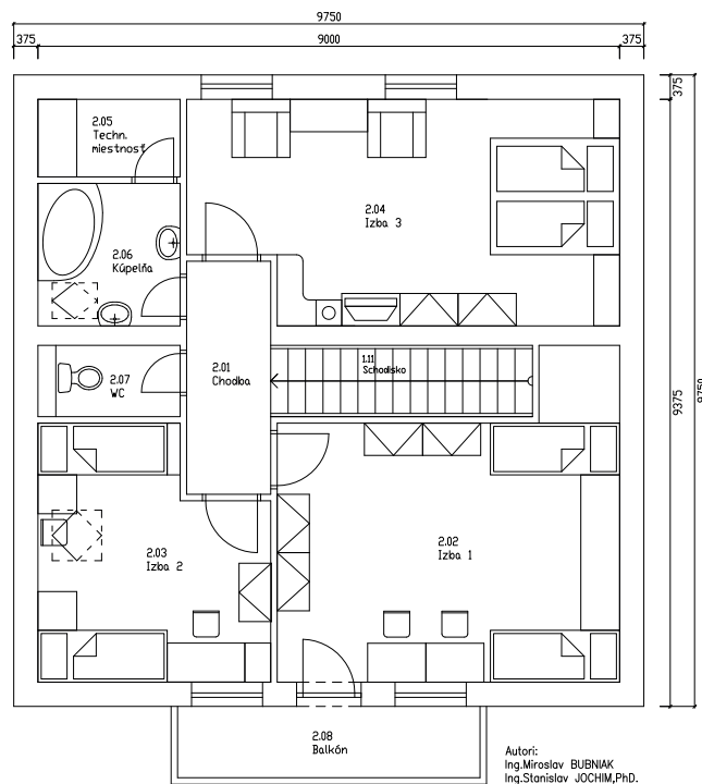
Obr.2: Pôdorys 2NP analyzovaného domu
