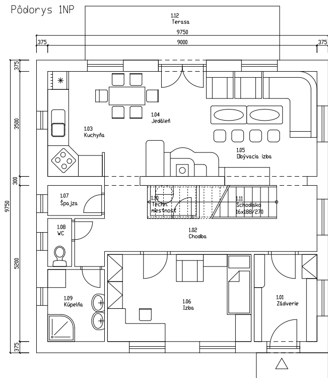
Obr.1: Pôdorys 1NP analyzovaného domu
